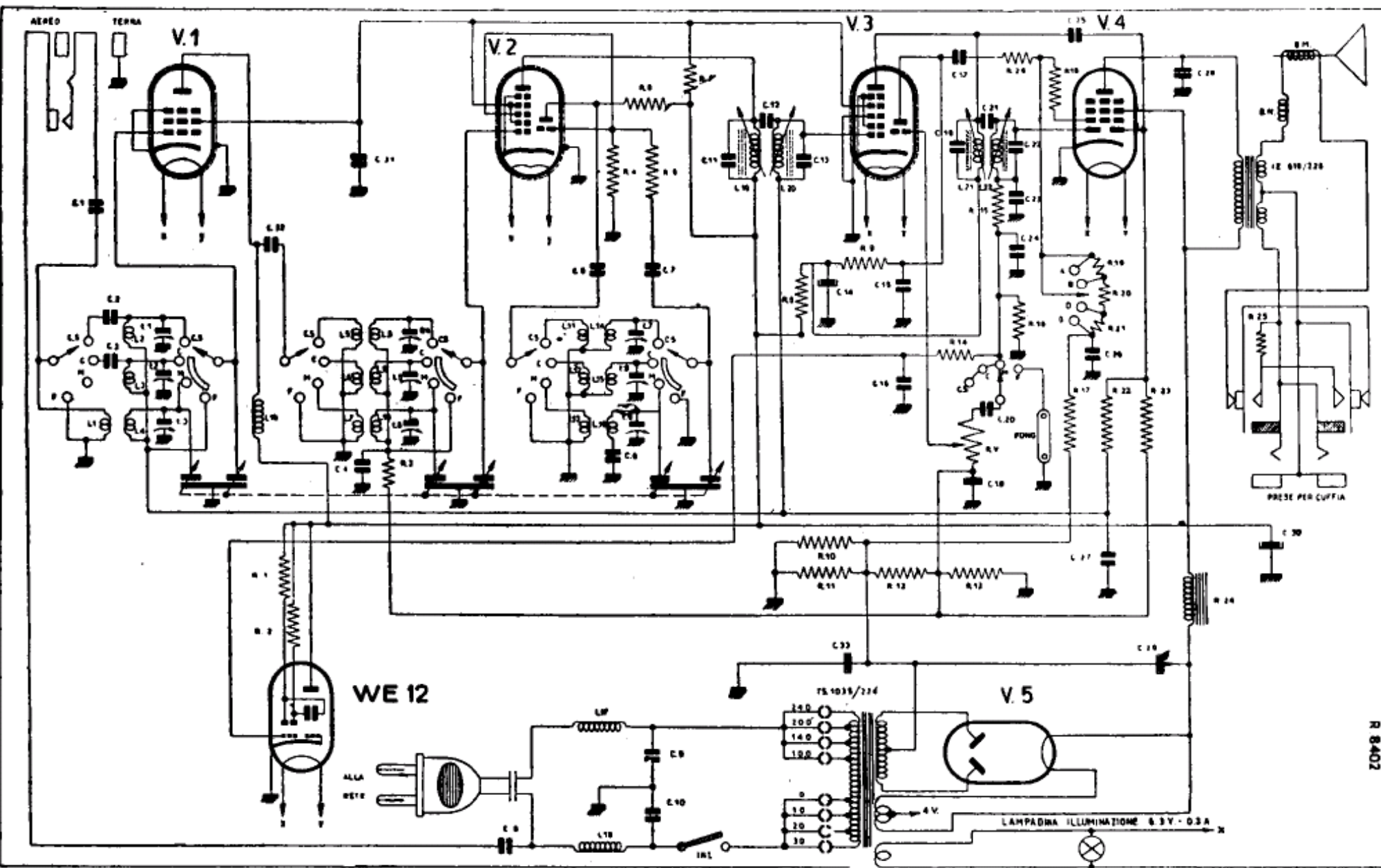
PHONOLA (S. A. FIMI). — Mod. 559-581 e 582. — Media frequenza: 470 kHz. VALVOLE: V1 = 6K7G; V2 = ECH4; V3 = ECH4; V4 = EBL1; V5 = 5Y3G.
